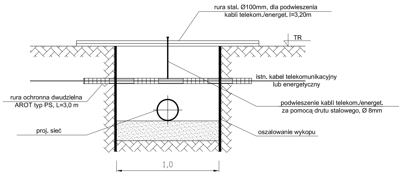
SCHEMAT ZABEZPIECZENIA KABLI W MIEJSCU SKRZYŻOWANIA Z PROJEKTOWANYM KANALEM SANITARNYM LUB PRZYŁĄCZAMI
