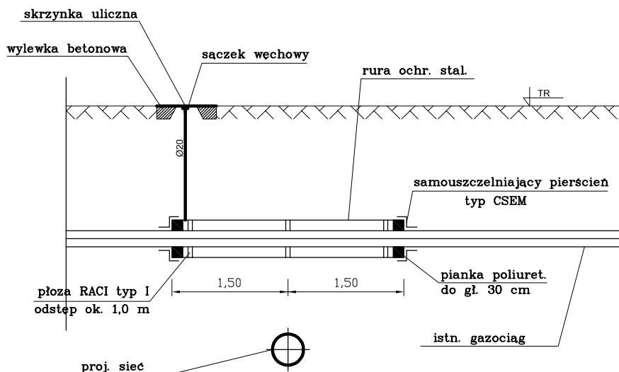
SCHEMAT ZABEZPIECZENIA GAZOCIĄGU W MIEJSCU SKRZYŻOWANIA Z PROJEKTOWANYMI PRZYŁĄCZAMI KANALIZACJI SANITARNEJ
